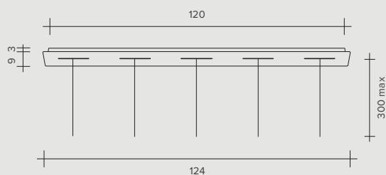
5xG9 max 28W - 230V
