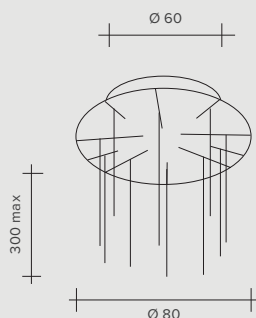
10x G9 max 28W - 230V
