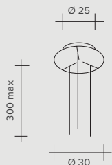
3xG9 max 28W - 230V
