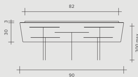
5xG9 max 28W - 230V
